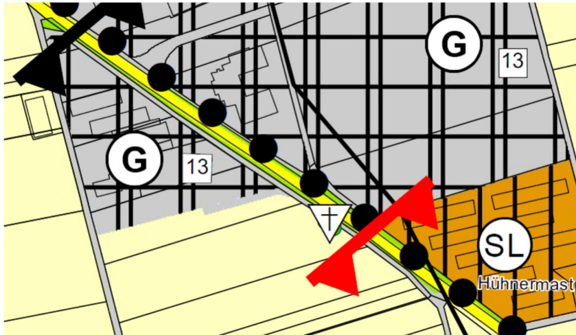
Flächennutzungsplan – Bestands-Ausschnitt
